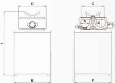
Vibratore circolare da 5-7-11-16 litri 2 velocità 5-7-11-16 liter circular vibrator by two speed
